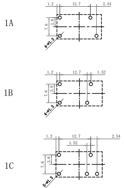
安装孔尺寸图 (底视图)
