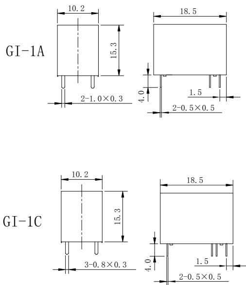
外形图
