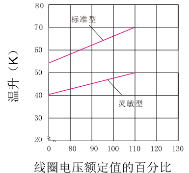
线圈温升
