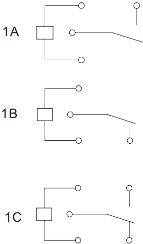
接线图
