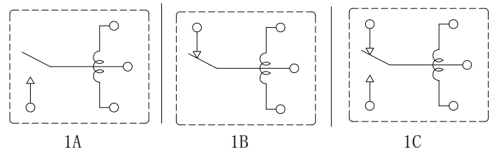
接线图
