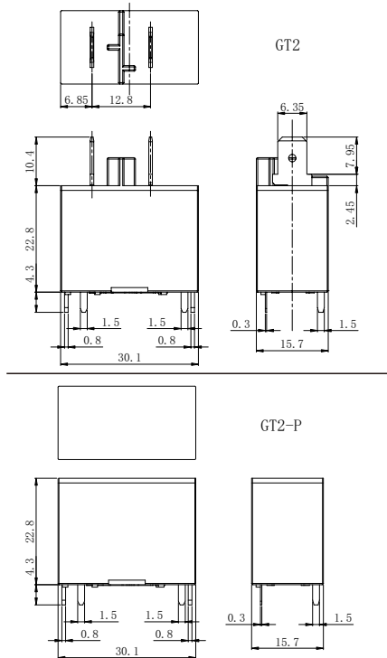
外形图
