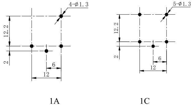
安装孔尺寸图
